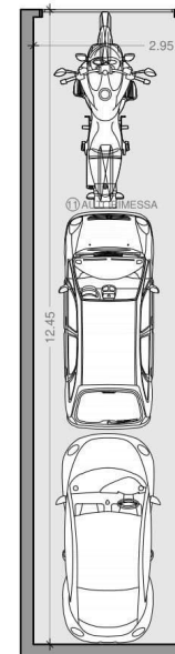
PLANIMETRIA PIANO INTERRATO
