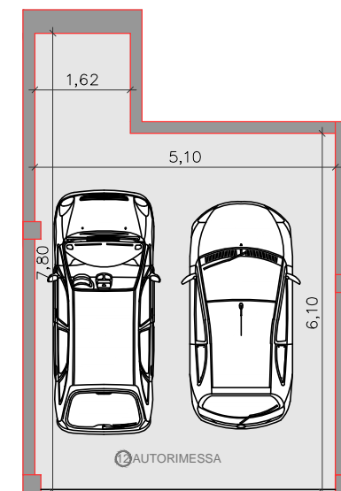
PLANIMETRIA PIANO INTERRATO
