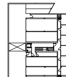
PLANIMETRIA GENERALE PIANO INTERRATO
