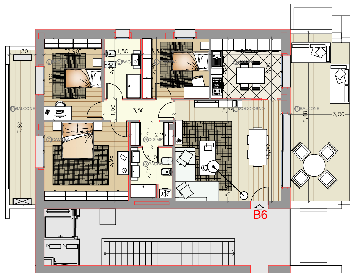
PLANIMETRIA PIANO SECONDO
