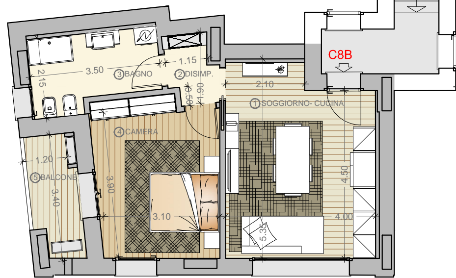
PLANIMETRIA PIANO PRIMO
