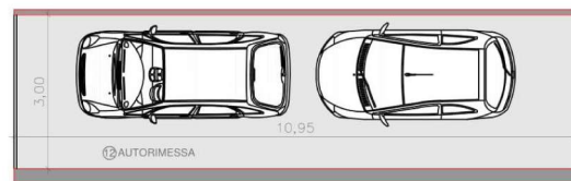
PLANIMETRIA PIANO INTERRATO
