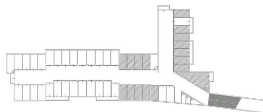
PLANIMETRIA GENERALE PIANO INTERRATO
